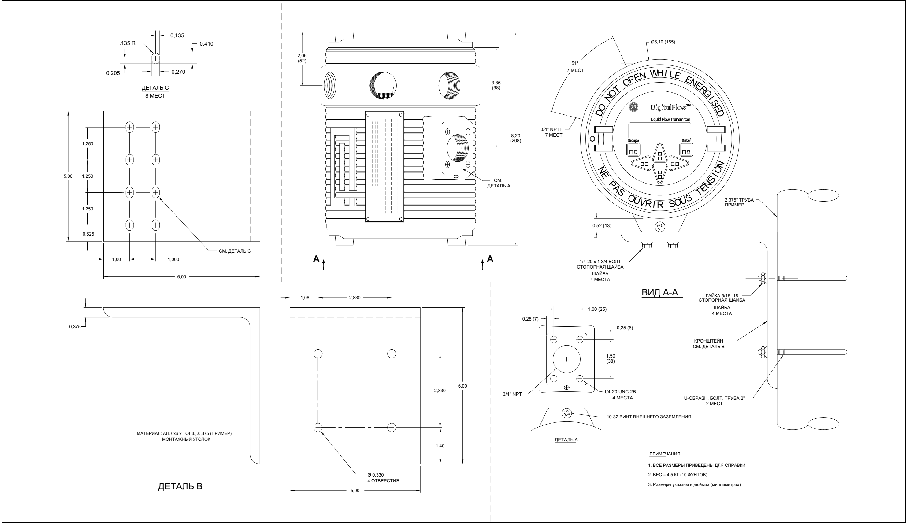
Рис. 6: Прямоугольный монтажный кронштейн — Электронный блок (чертеж № 712-1317)
