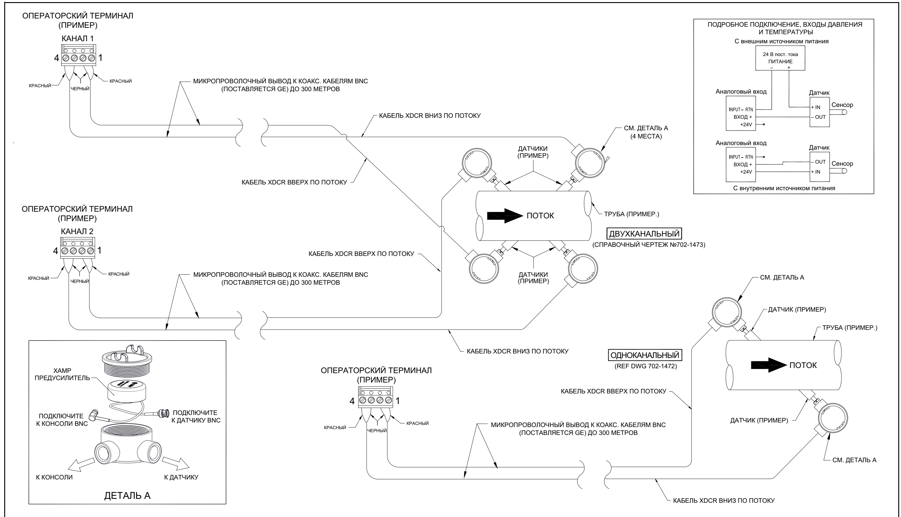
Рис. 10: Электромонтажная схема — датчики с локальным предусилителем (ХАМР)
