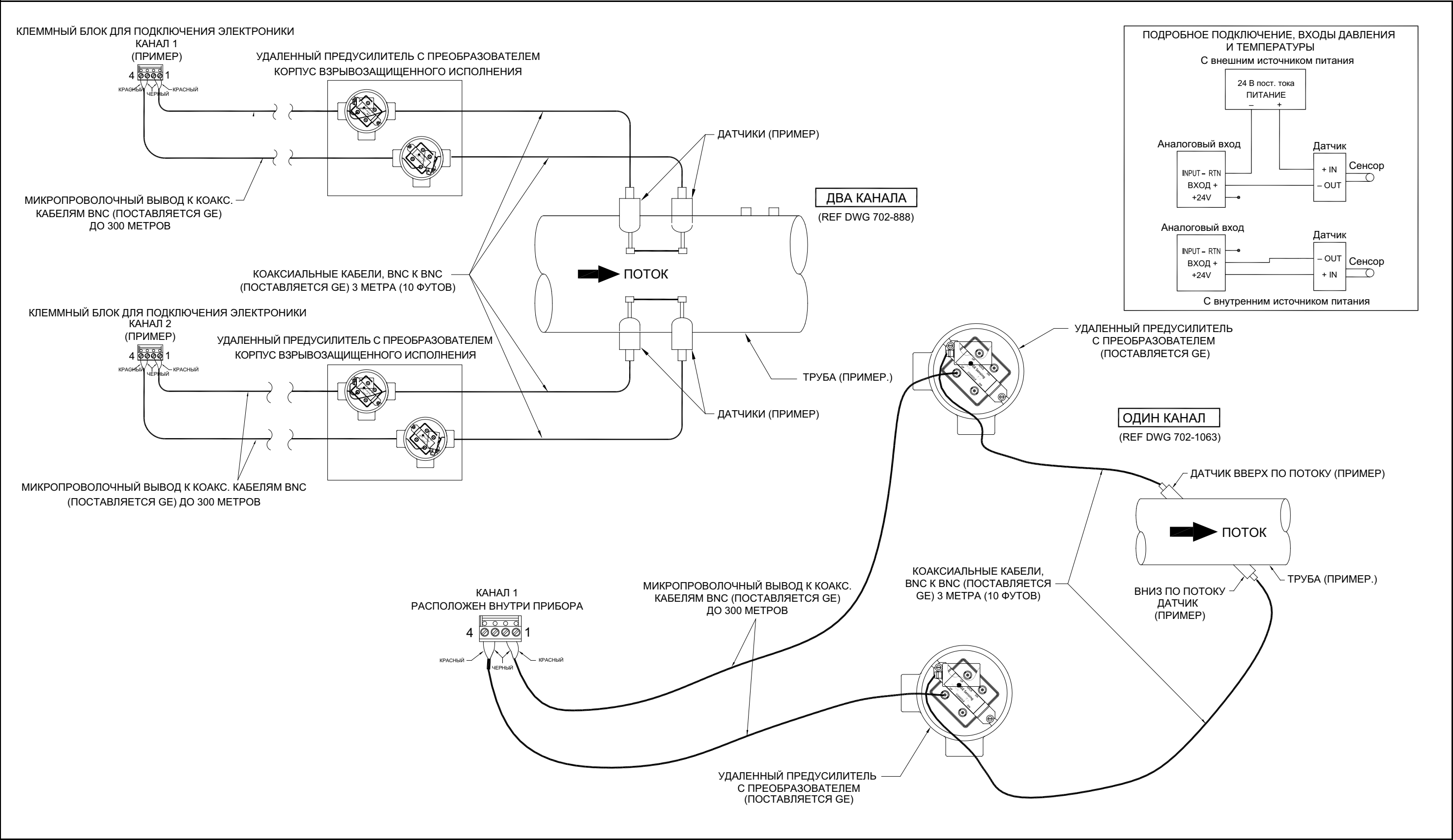
Рис. 9: Электромонтажная схема — датчики с удаленным предусилителем (PRE868) и трансформатором
